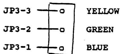
Fig. 5 - S1 Wiring
